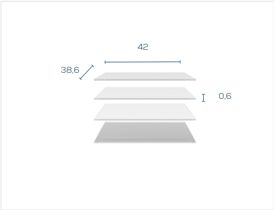
Glaseinlegeböden 9822
