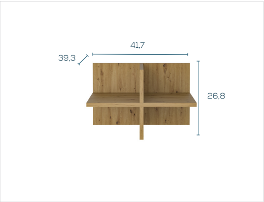
Einsatz 9921
